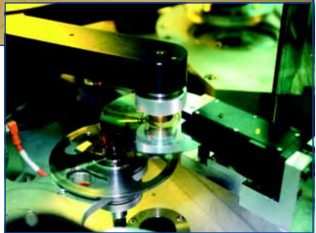
Neues Inline Meßsystem für SPACELINE Anlagen
