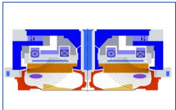
Prinzip der Smart Cathode®: Sputtern am Außenradius
