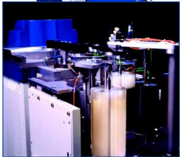
SINGULUS III DVD Metallizer mit integriertem Handling-System
