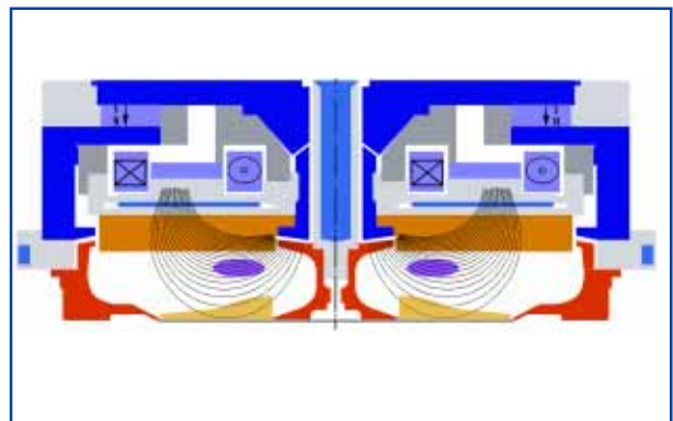
Prinzip der Smart Cathode®: Sputtern am Innenradius
