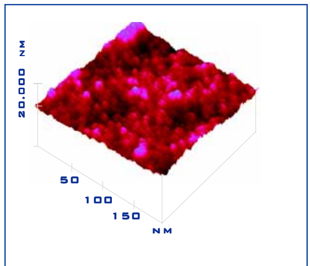
AFM-Untersuchung einer Silizium-Schicht mit geringer Rauhtiefe für DVD 9
